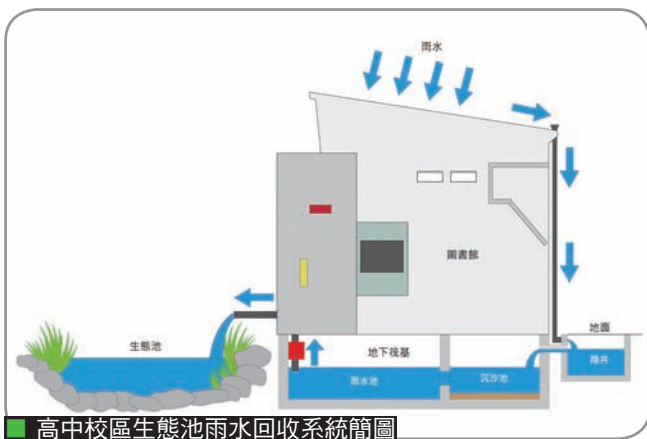
高中校區生態池雨水回收系統簡圖
